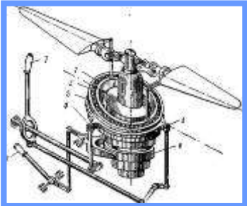
Автомат перекося Юрьева
