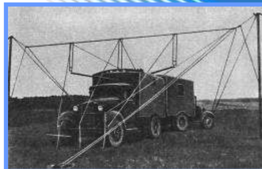
Передающая и приемная станции РЛС системы РУС-1 «Ревень»
